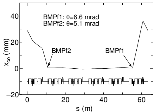
図 5：入射バンプ軌道。
