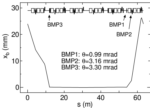
図 9：出射バンブ軌道。
