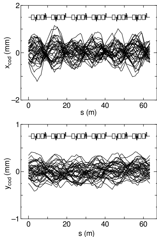
図 1-(b): 補正後の残留閉軌道誤差。
